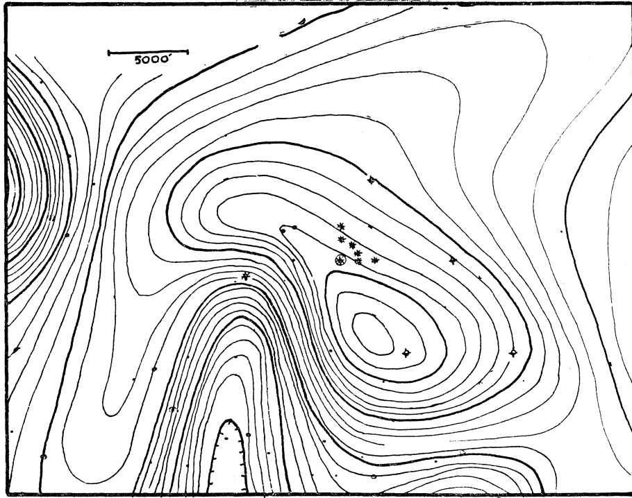
Şekil 117 ___W14 Goose gaz sahasına ait sismik refleksiyon konturlar haritası ve âero.manyetik harita
