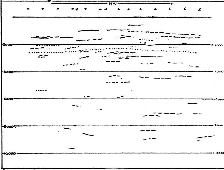
Şekil : 16 - Wild Goose gaz sahasına ait sismik refleksiyo kesiti
