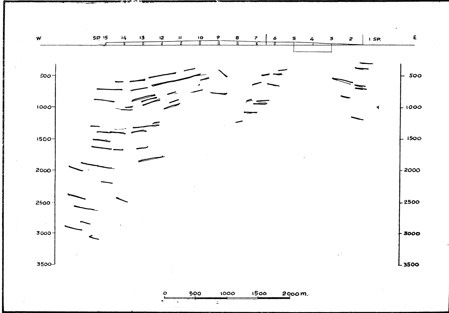
Şekil:14 – Sismik refleksiyon kesiti
